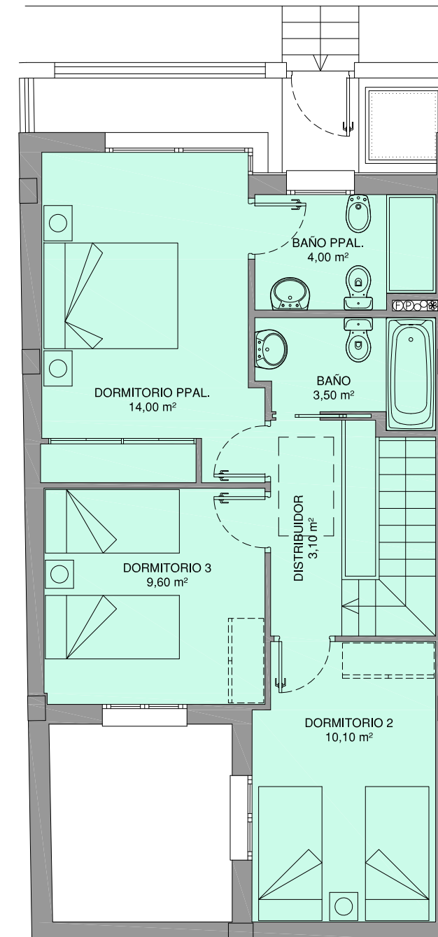
PLANTA ALTA
