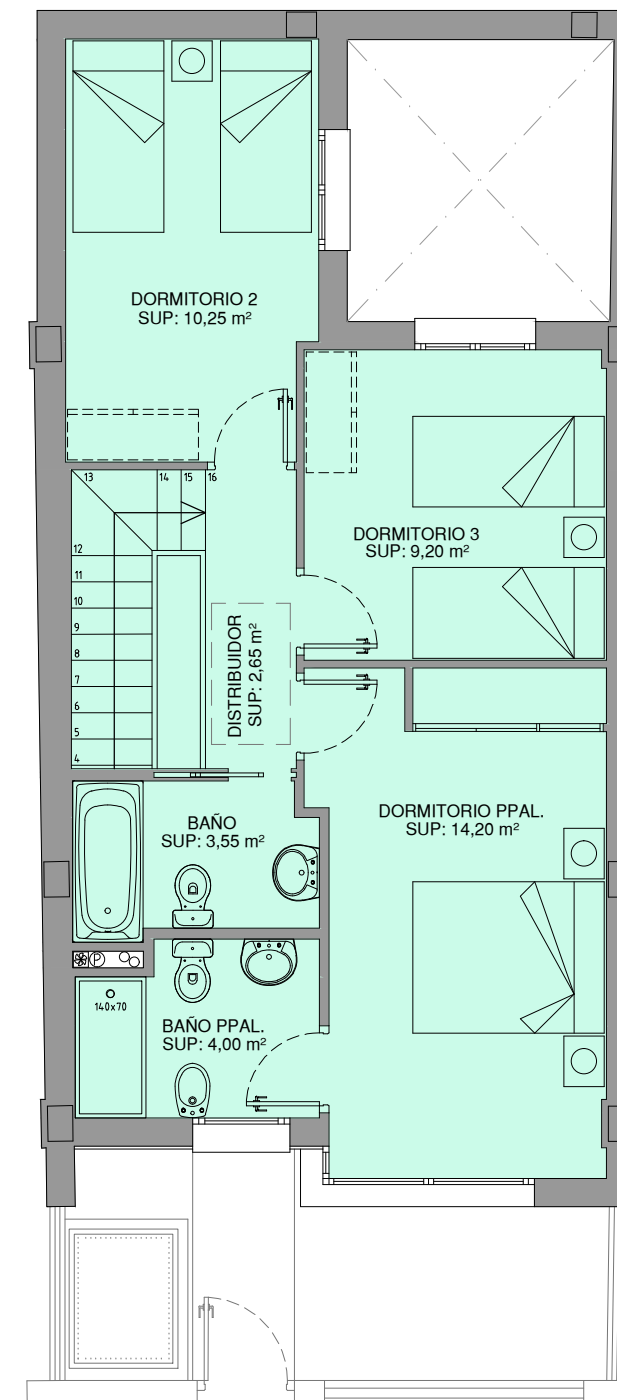
PLANTA ALTA
