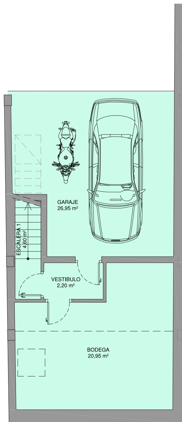
PLANTA SEMISOTANO
