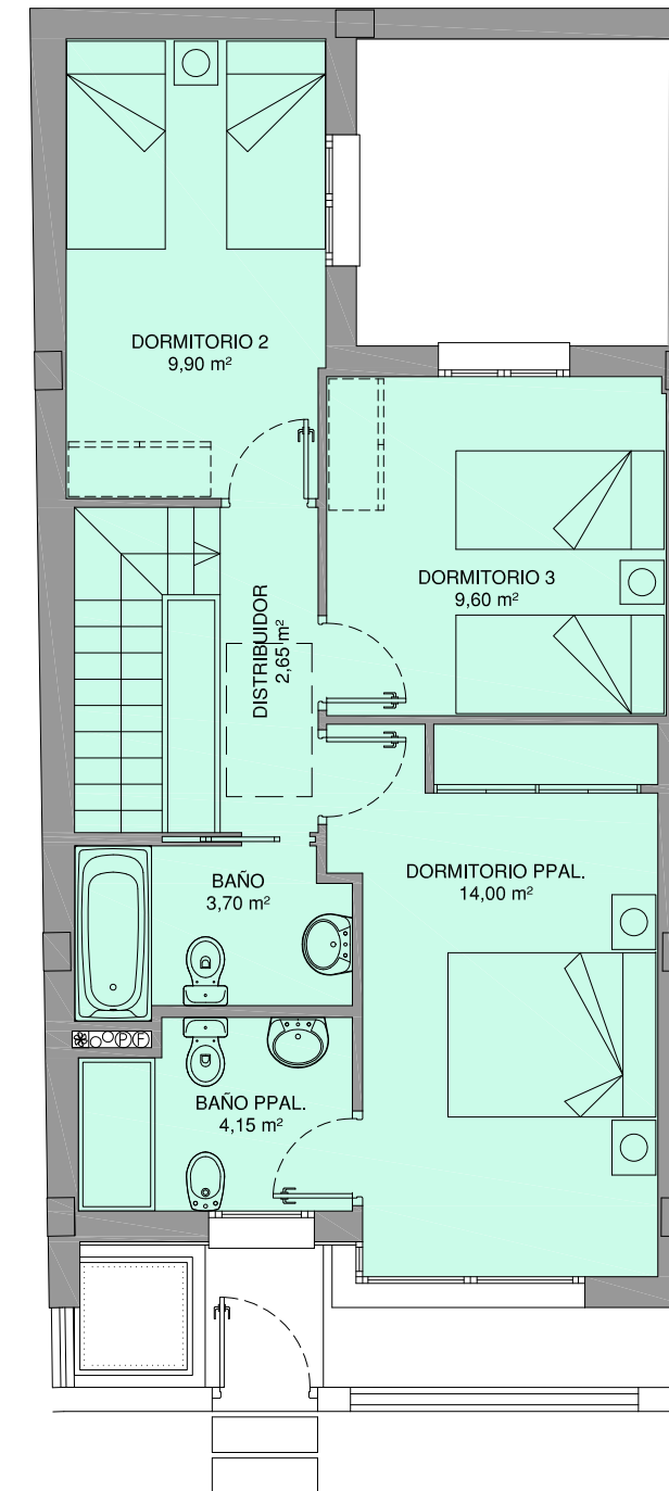
PLANTA ALTA
