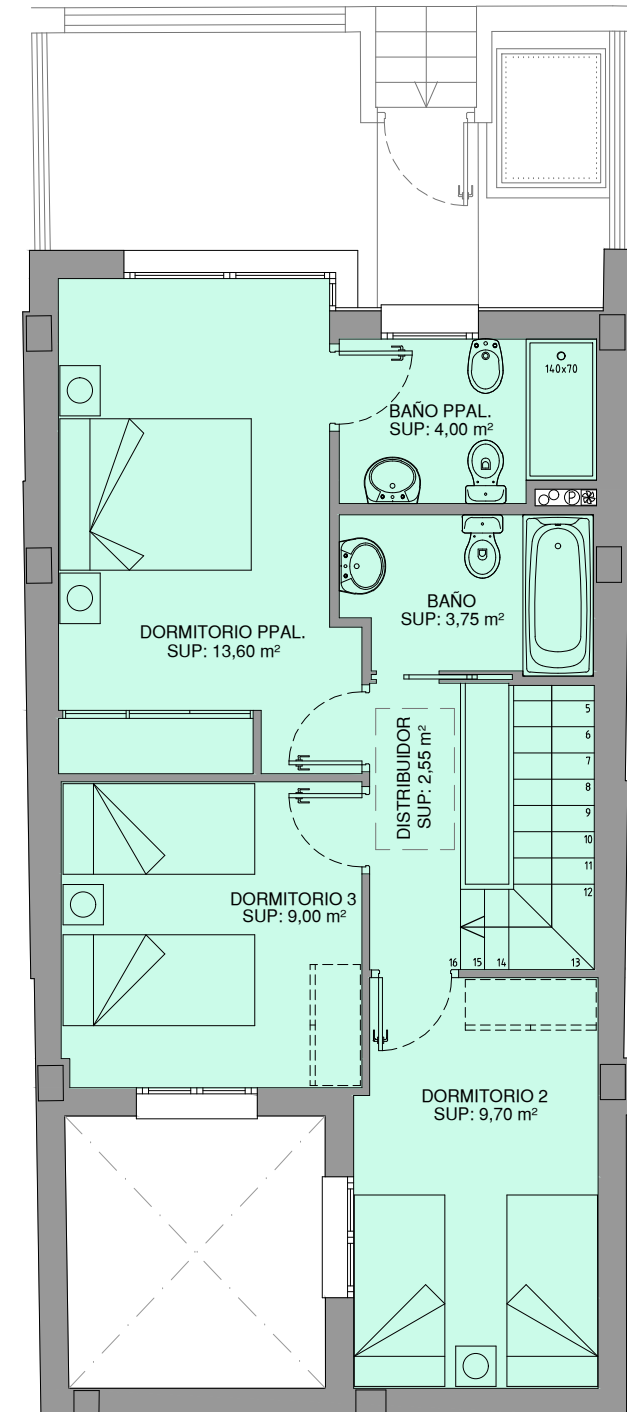
PLANTA ALTA
