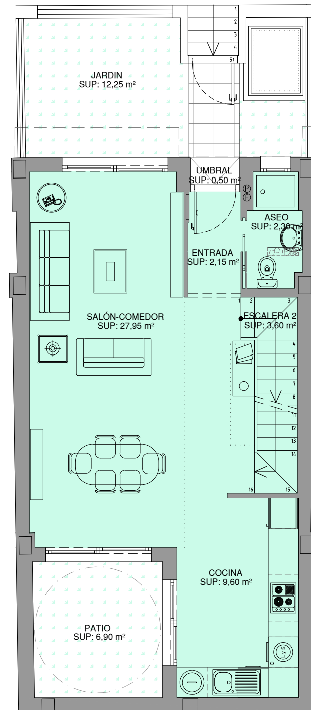
PLANTA BAJA
