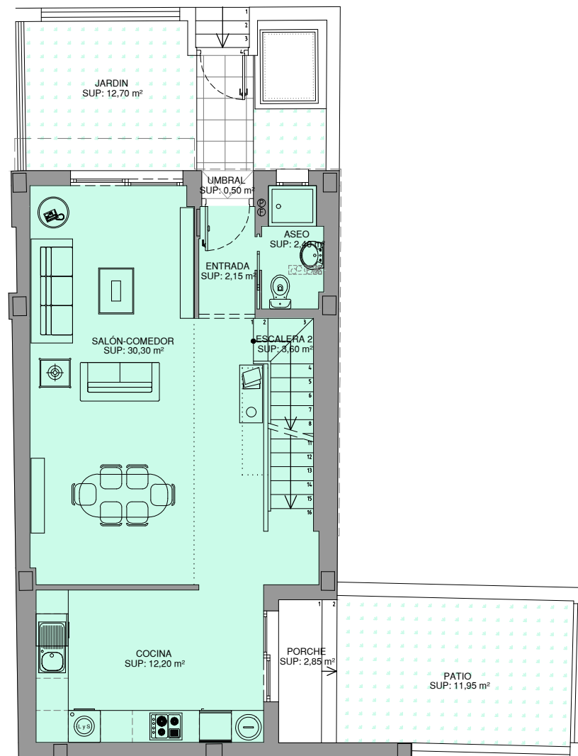
PLANTA BAJA
