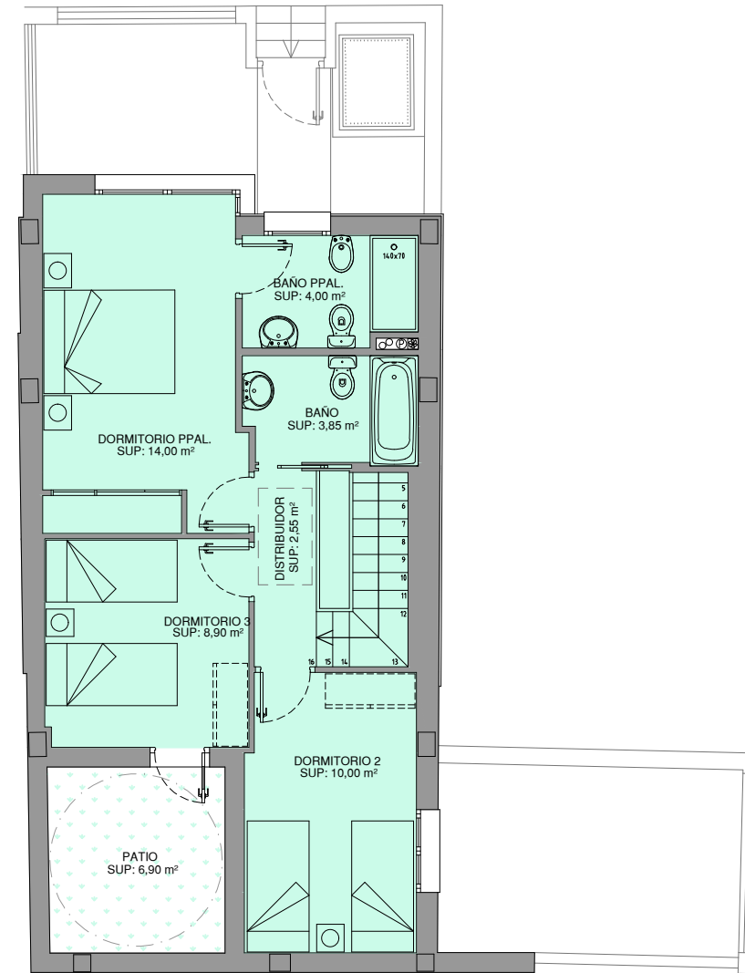
PLANTA ALTA
