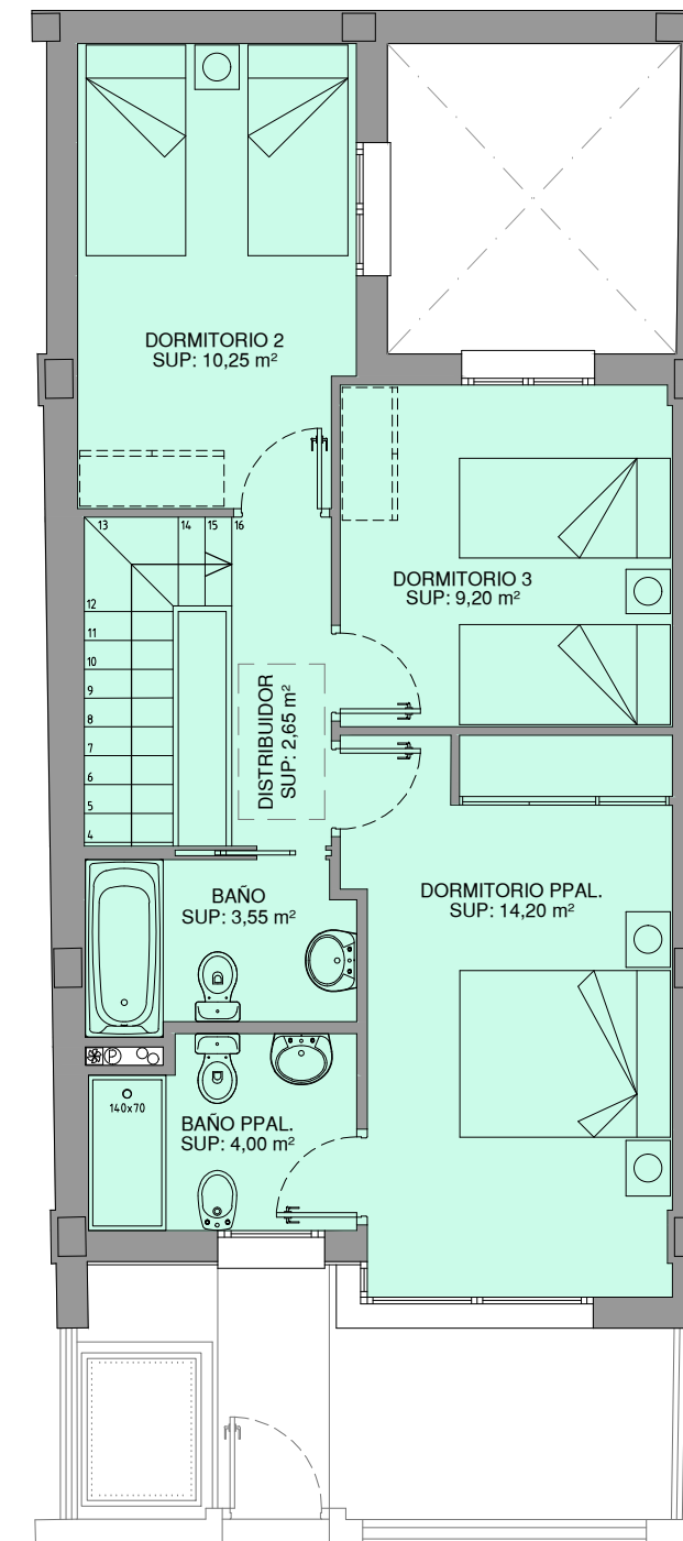
PLANTA ALTA
