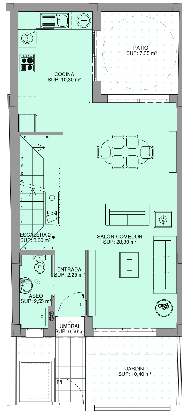
PLANTA BAJA
