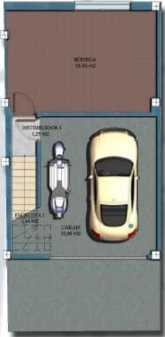
P. SEMISOTANO
